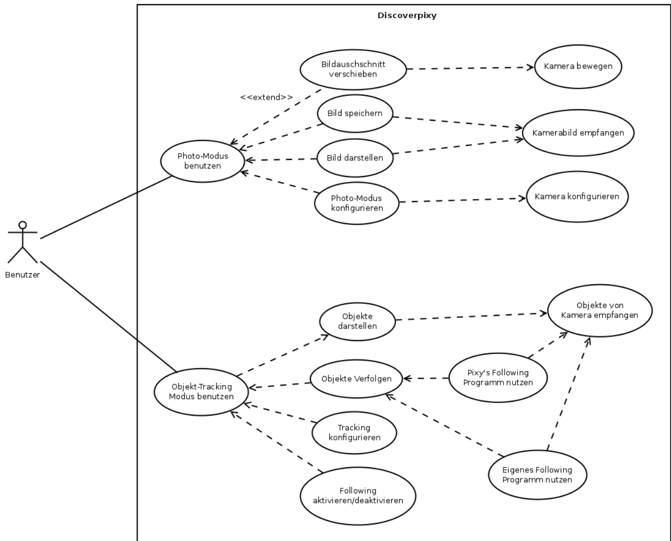
Illustration 2: Anwendungsfalldiagramm
