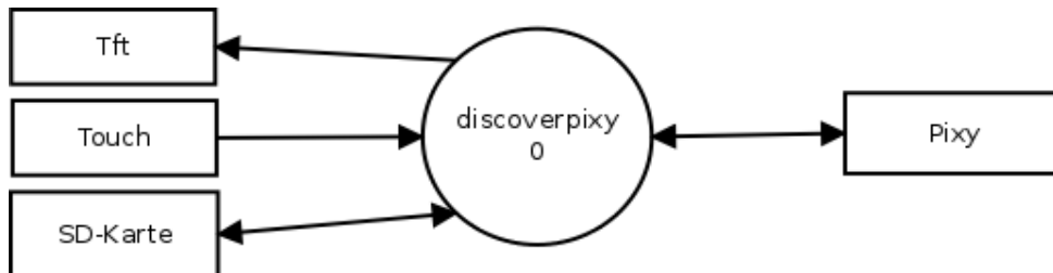
Illustration 1: Kontextdiagramm
